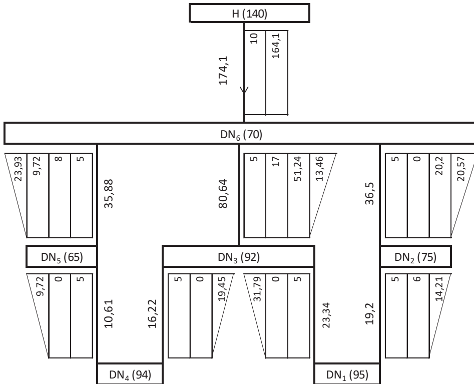
Şekil 4. İki gözülü şebekenin şematik ÖN yöntemi ile çözülmesi.
