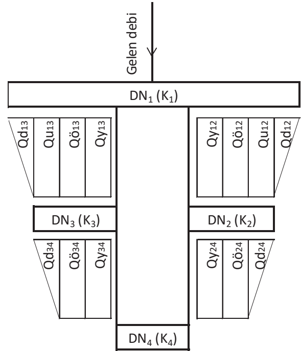
Şekil 2. Şematik ÖN yöntemi tipik şebeke gözü çizimi.
