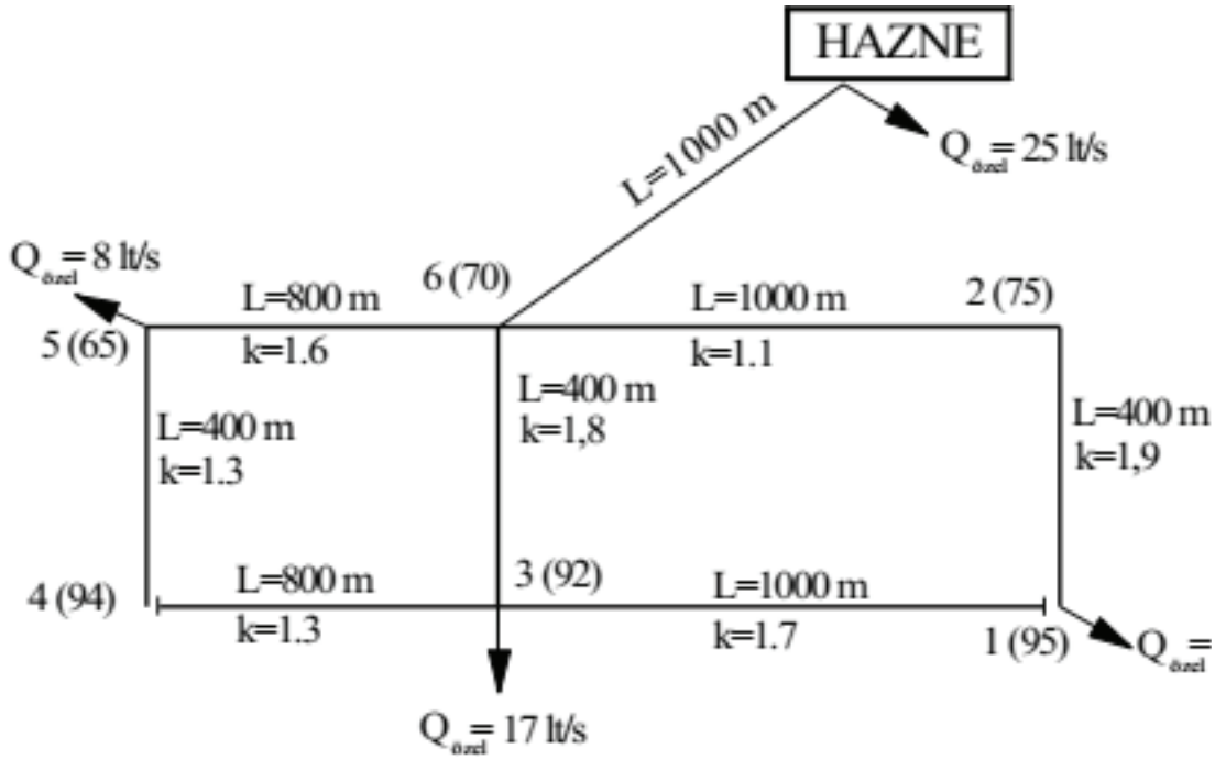
Şekil.3 İki gözlü örnek şebeke.
