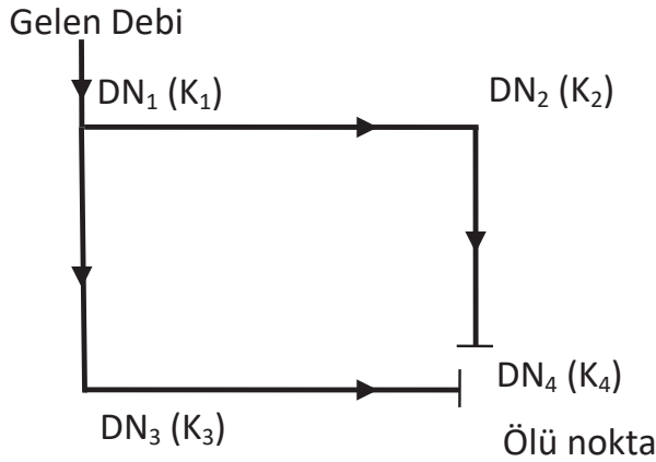
Şekil 1. Tipik şebeke gözü çizimi.
